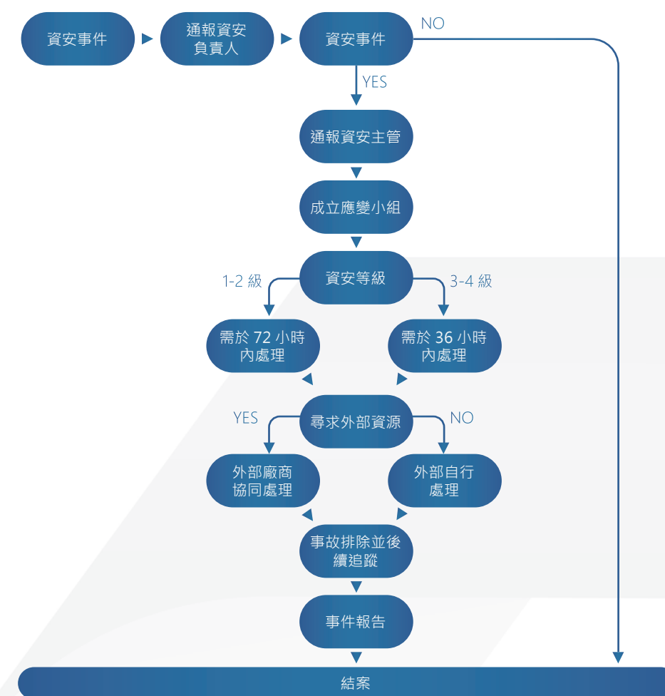
資安通報流程圖
