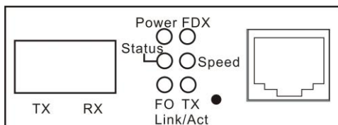
図 1. 2芯ファイバタイプの前面パネル
